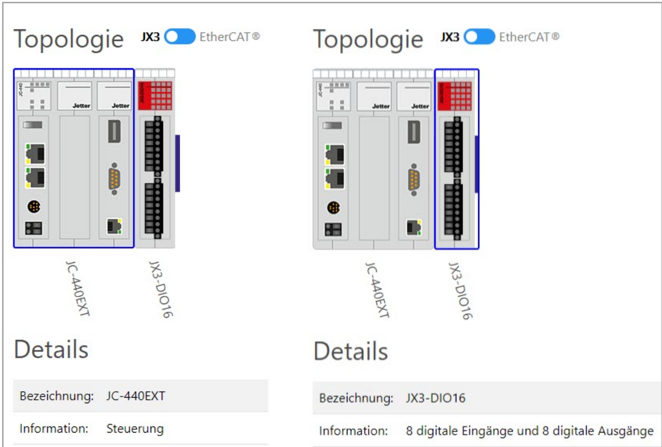
Abb. 12: Seite Topologie mit Informationen zur Hardware, die via JX3-Bus verbunden ist.
