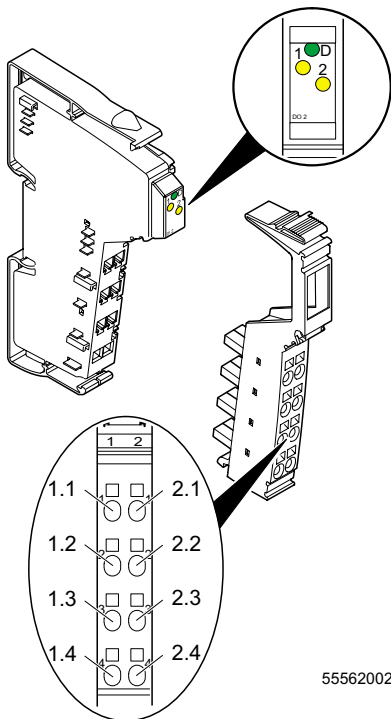
Bild 2 IB IL 24 DO 2 mit zugehörigem Stecker
