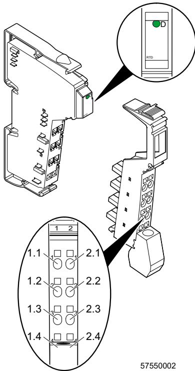
Bild 2 IB IL TEMP 2 RTD mit zugehörigem Stecker
