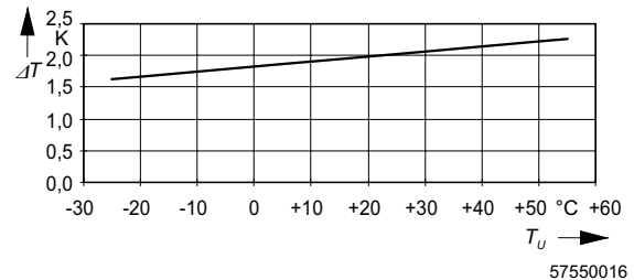
Bild 17 Systematischer Temperaturmessfehler \Delta T in Abhängigkeit von der Leitungstemperatur T_U
