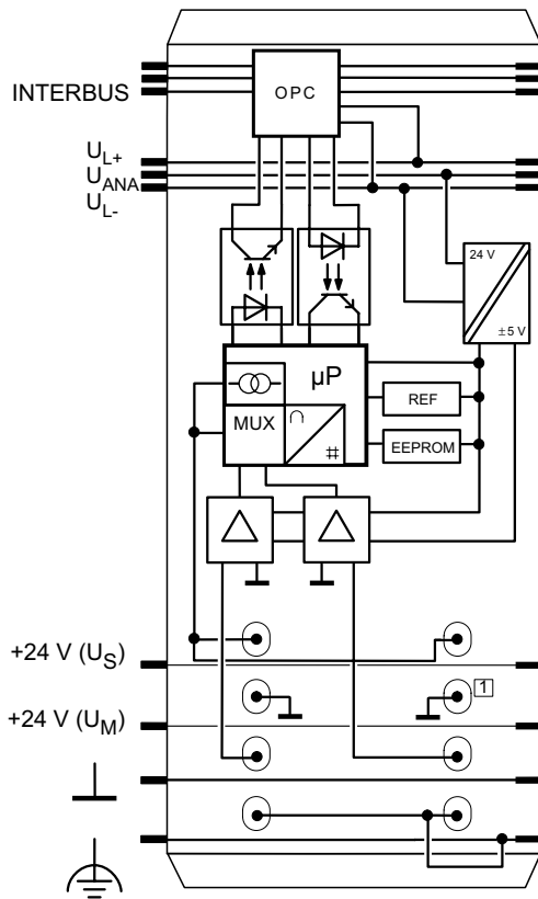
Bild 3 Interne Beschaltung der Klemmpunkte
