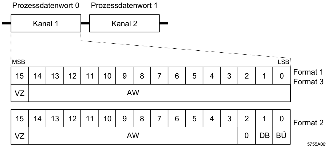
Bild 8 Reihenfolge der Prozessdaten-Eingangsworte im INTERBUS-Ring und Darstellung der Bits des ersten Prozessdatenwortes in den verschiedenen Formaten
