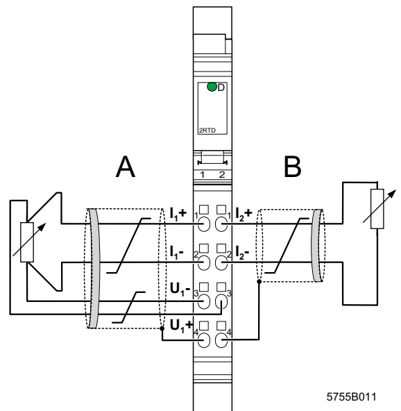
Bild 6 Anschluss von Sensoren in 4- und 2-Leitertechnik mit Schirmanschluss
