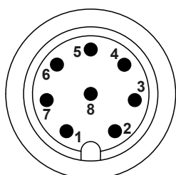
Fig. 6: Spina M12
