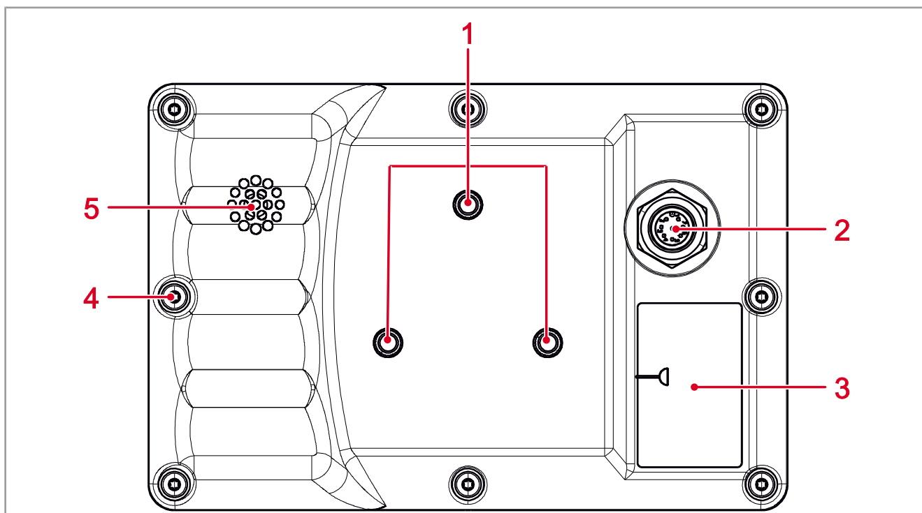
Fig. 2: Parte posteriore del dispositivo di comando
