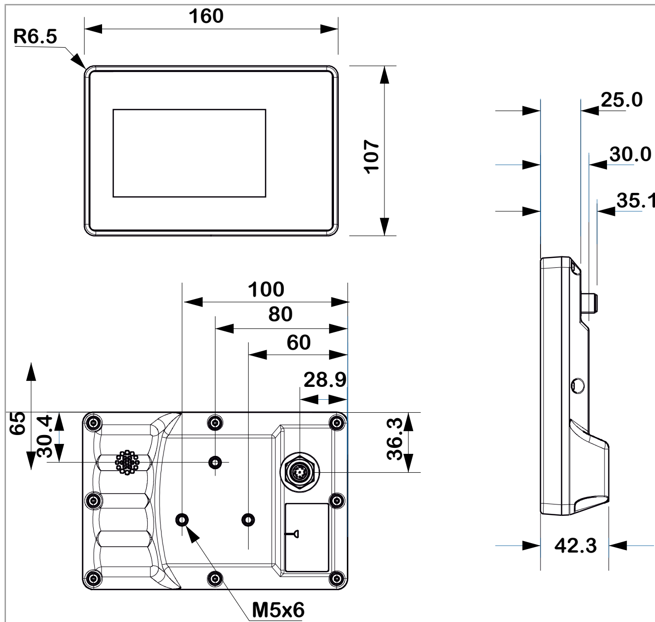
Fig. 4: Dimensioni in mm
