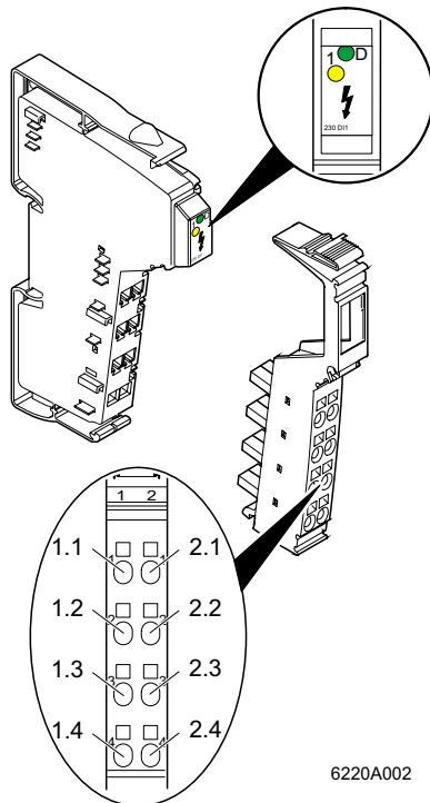
Figure 2 IB IL 230 DI 1 with the appropriate connector
