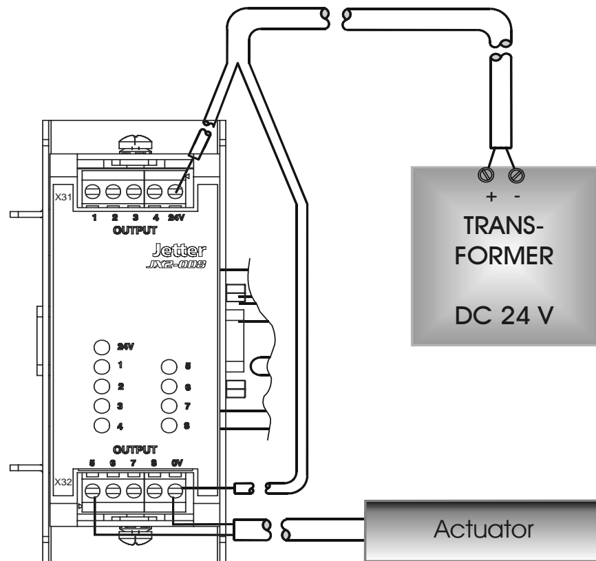
Fig. 5: Example: Output Wiring of a JX2-OD8 Module
